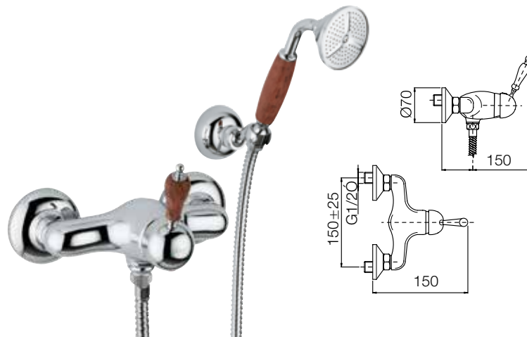
6000-5 Monocomando doccia esterno con doccia duplex Single lever shower mixer with shower duplex
