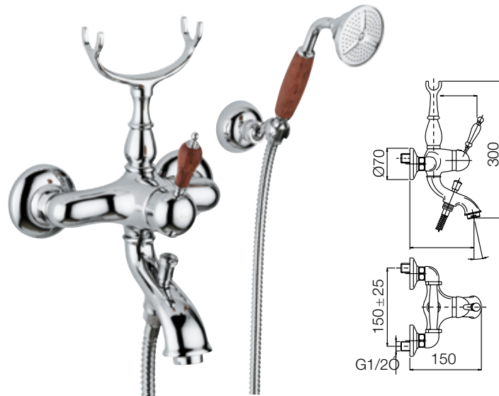
6000-3 Monocomando vasca esterno con doccia duplex Single lever bath mixer with shower duplex
